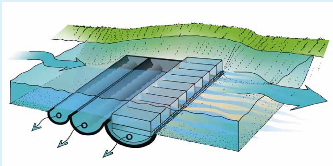
Afb. 1: Schematisch overzicht van de Mudtrap.
